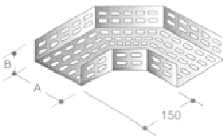
Curva Horizontal 90°
